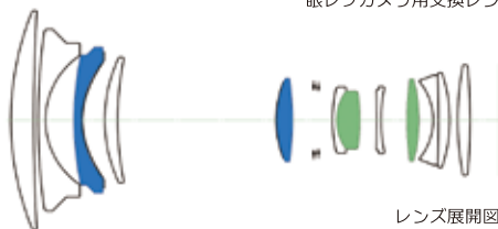
レンズ展開図
